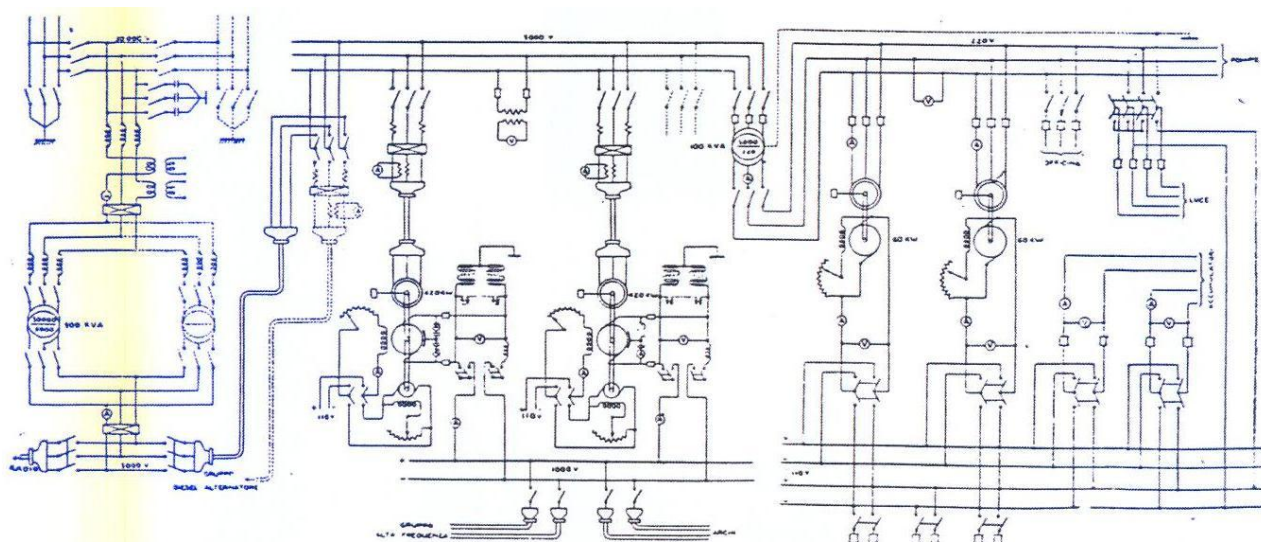
Fig. 7. — Schema elettrico principale.
