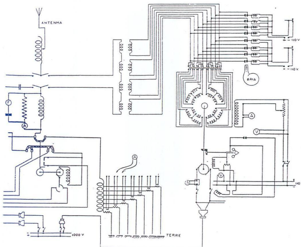
Fig. 13. — Schema dell'impianto dell'alternatore ad alta frequenza.
